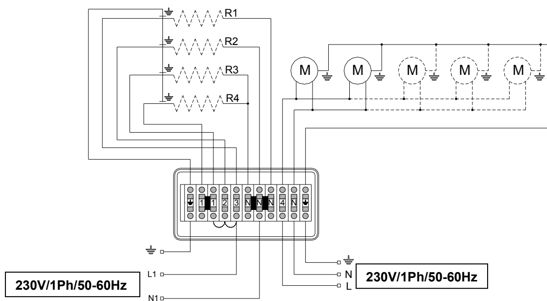
Schema elettrico con alimentazione resistenze a 230V/1Ph/50-60Hz
