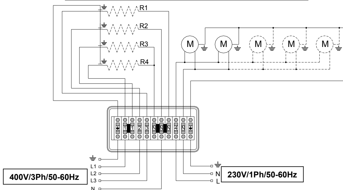
Schema elettrico con alimentazione resistenze a 400V/3Ph/50-60Hz
